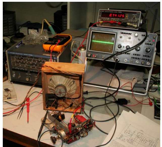
Het toestel omringt door de testapparatuur (ook van Philips)
