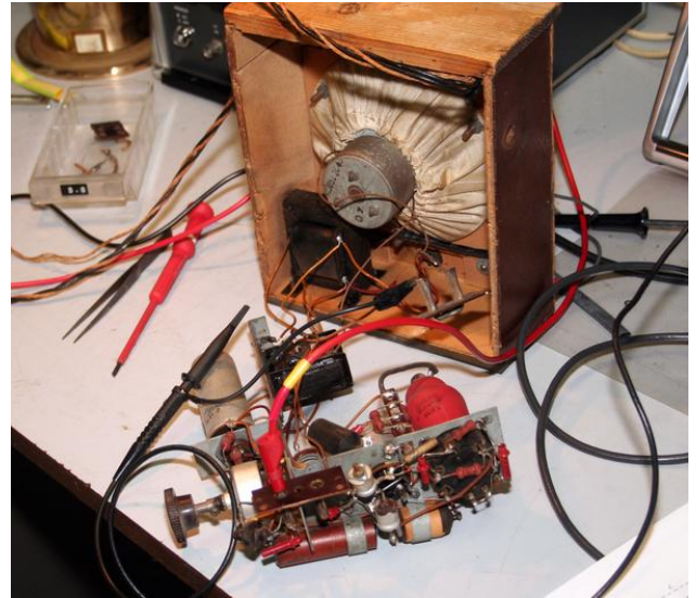
De Luistervink met het chassis uit de kas genomen. Rechts de (rode) buis type ECF1
